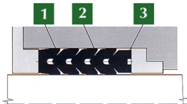
1 – Opěrný kroužek 2 – Manžeta ševron 3 – Přítlačný kroužek
